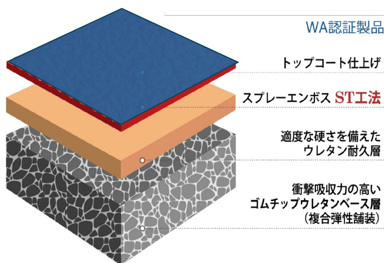
■陸上トラックの断面構成
